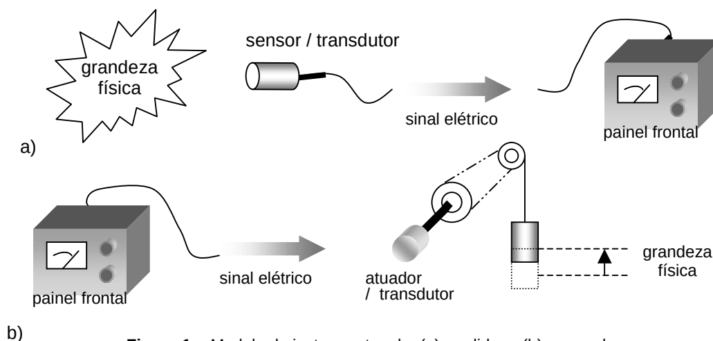
Figura 1 - Modelo de instrumentos de (a) medida e (b) comando.
