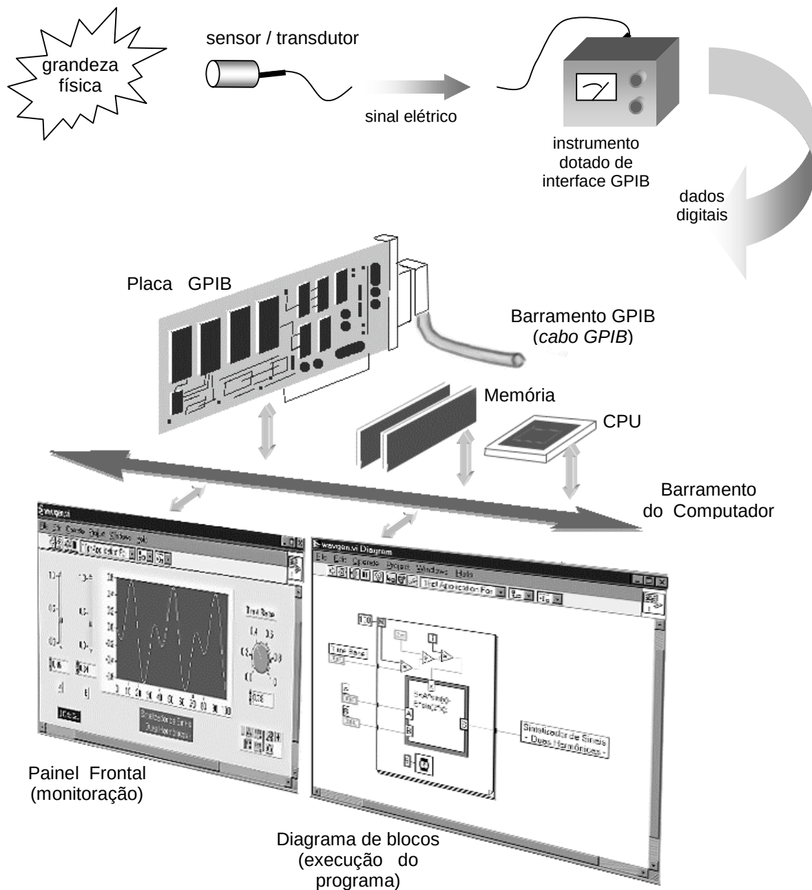
Figura 3 - Estrutura de um instrumento virtual
