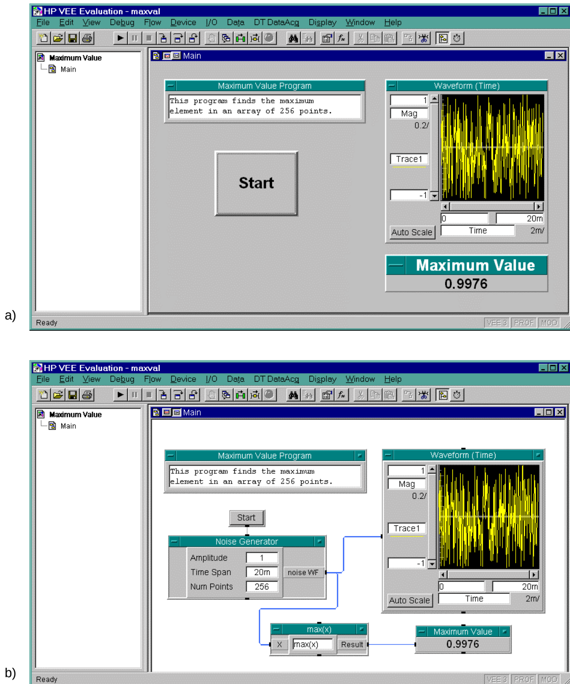
Figura 5 - Solução implementada com HP-VEE.
